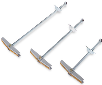
Tuimelanker M10 inclusief verdiepingsring 250-350-450mm (109795 t/m 109797)
